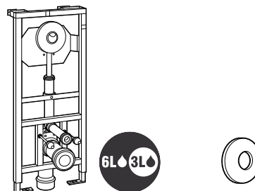
Duplo WC Fluxor
