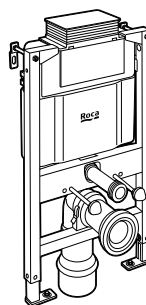
Duplo WC bajo ventana
